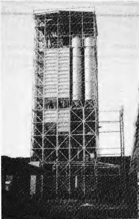
Trockenbaustoff-Mischanlage Berlin im Containerbausystem mit 2 Mischlinien Mischlinie I Stützenentleerung für Sackware Mischlinie II Ganzentleerung für lose Ware
